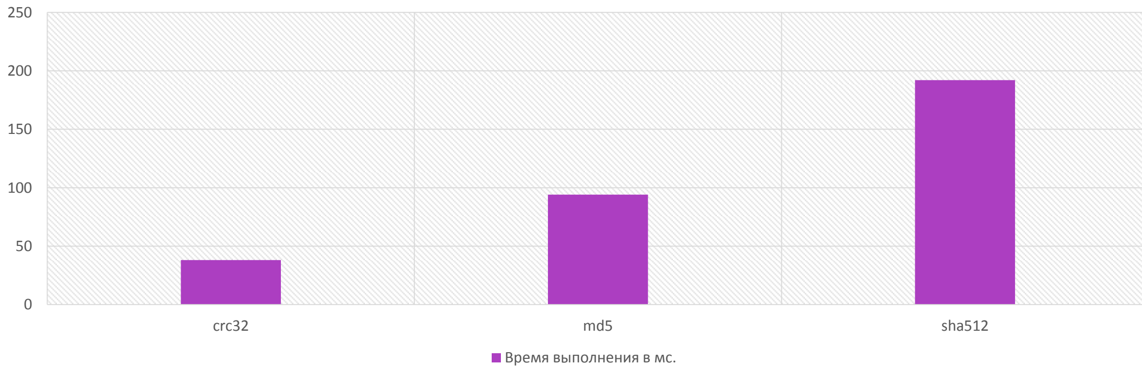
Время затраченное на создание хэша (50к вычислений)
