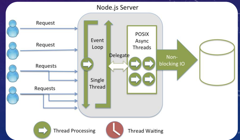
Структура Node.js
